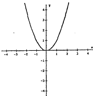
f(x) = x^2 Quadratic
